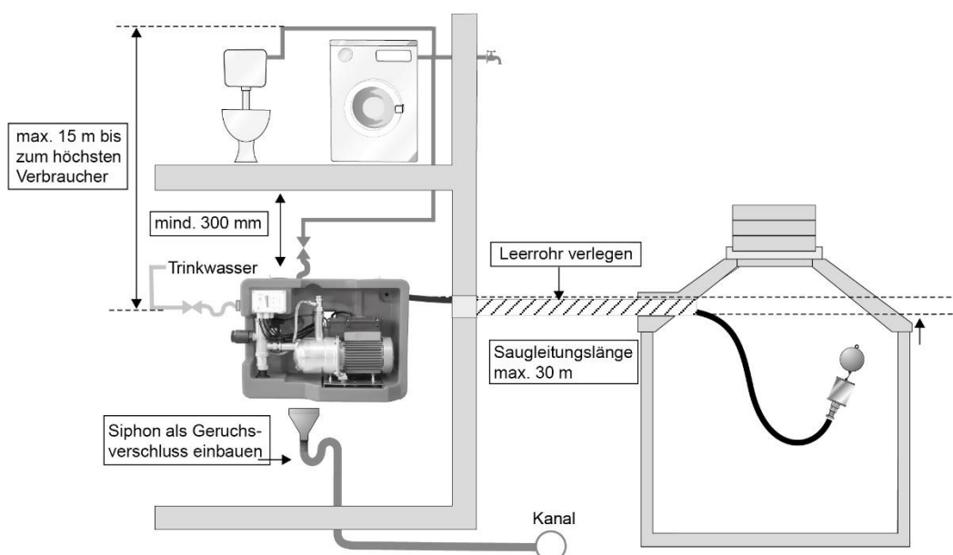
Hydraulischer Anschluss der RS 4500/6500
