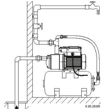
Fig. 2 Funzionamento in aspirazione Suction lift operation Saugbetrieb Fonctionnement en aspiration Funcionamiento en aspiración Sugande funktion Zuigsituatie Θέση λειτουργίας με κάθιση αναρρόφηση Работа выше уровня жидкости 负压水头工作
