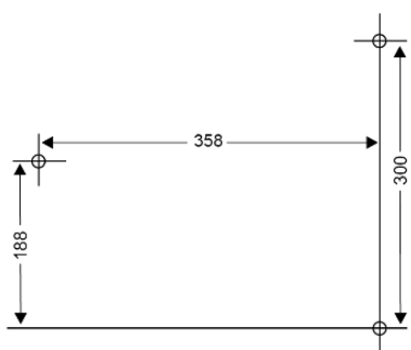
Lochschablone für Wandmontage RS 4500/6500
